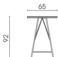
Seitenansicht TS65/TB65
